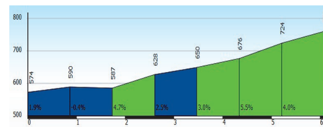
Pendenza media 3% circa (dislivello totale 185 metri circa)
