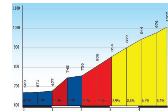
Pendenza media 7% (dislivello totale 340 metri circa)
