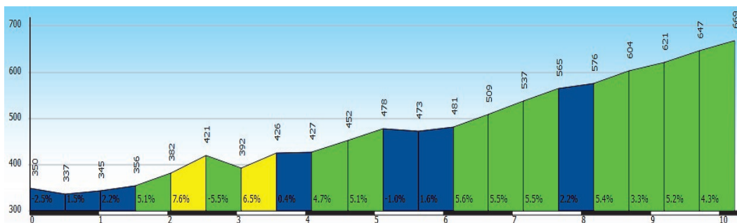
Pendenza media 3% circa (dislivello totale 315 metri circa)
