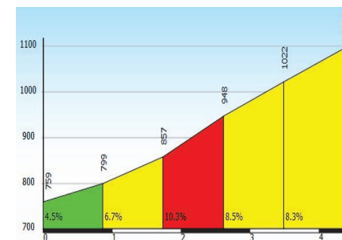
Pendenza media 8% (dislivello totale 335 metri circa)
